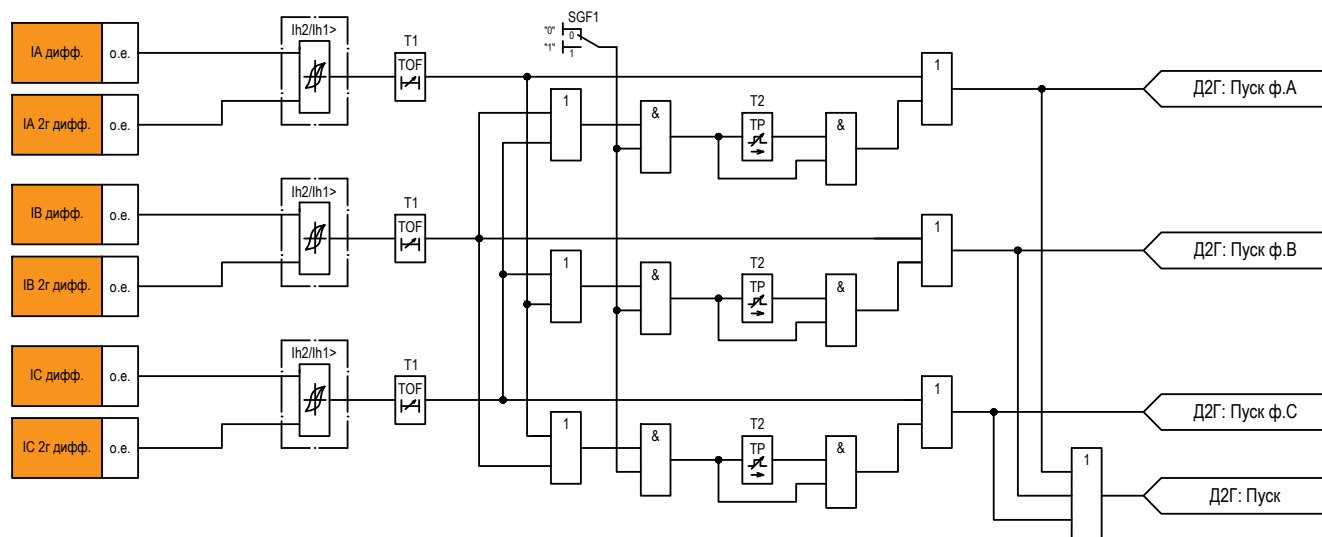
Рисунок 2.4 – Функциональная схема «Д2Г»
